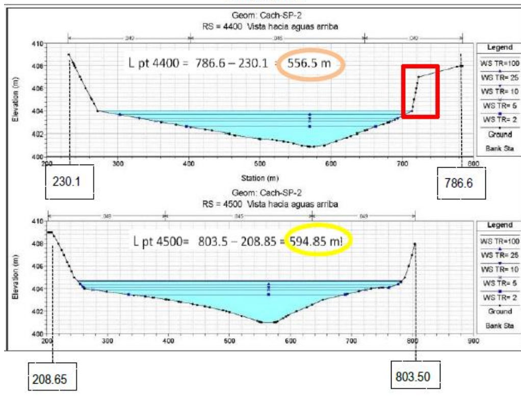
Figura 3 Mismas secciones extraídas del software de modelación hidráulica
