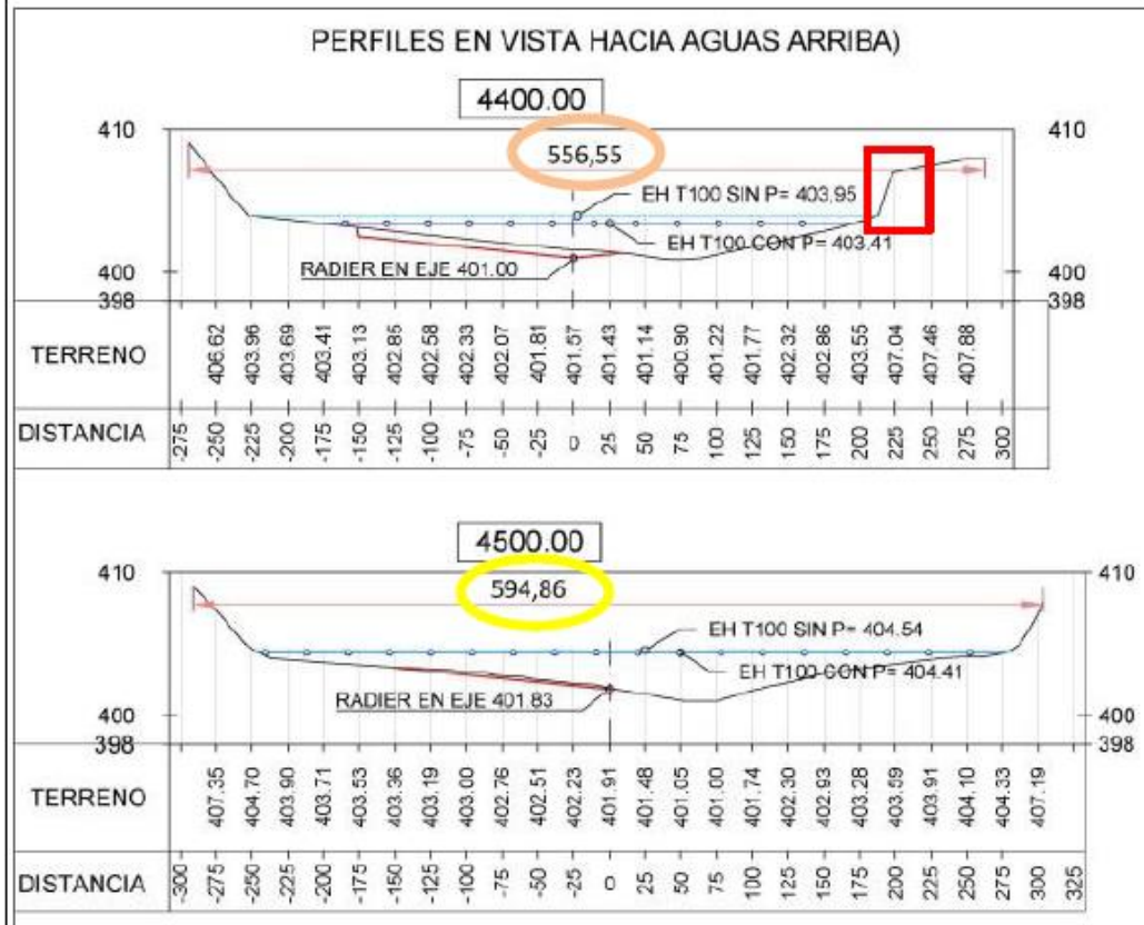
Figura 2 Perfiles Transversales PT 4400 y PT 4500 de Planos
