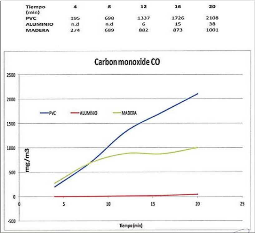
Fuente: Figura AC-38: Emisiones de Monóxido de Carbono (CO) del aluminio según ensayo de toxicidad de gases, Adenda Complementaria.
