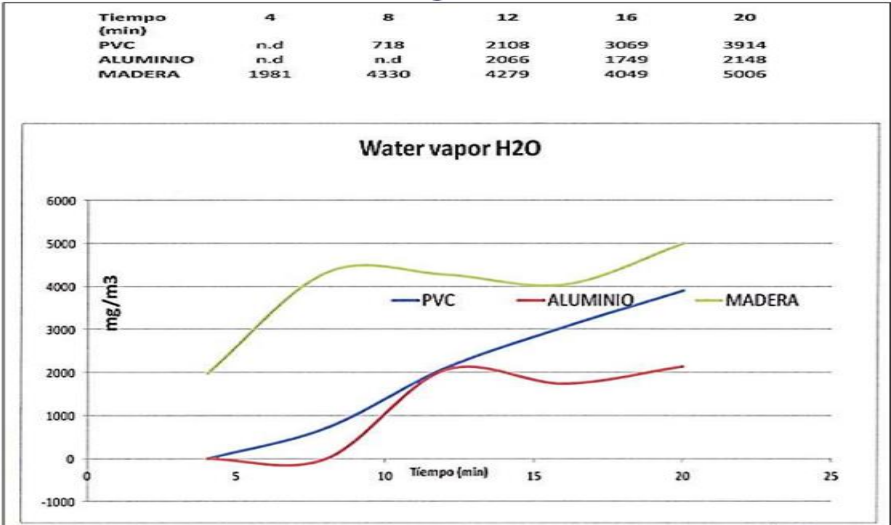
Figura: Emisiones de Vapor de agua (H 2 O) del aluminio según ensayo de toxicidad de gases
