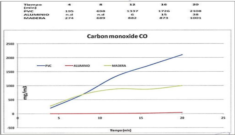
Fuente: Figura AC-38: Emisiones de Monóxido de Carbono (CO) del aluminio según ensayo de toxicidad de gases, Adenda Complementaria.
