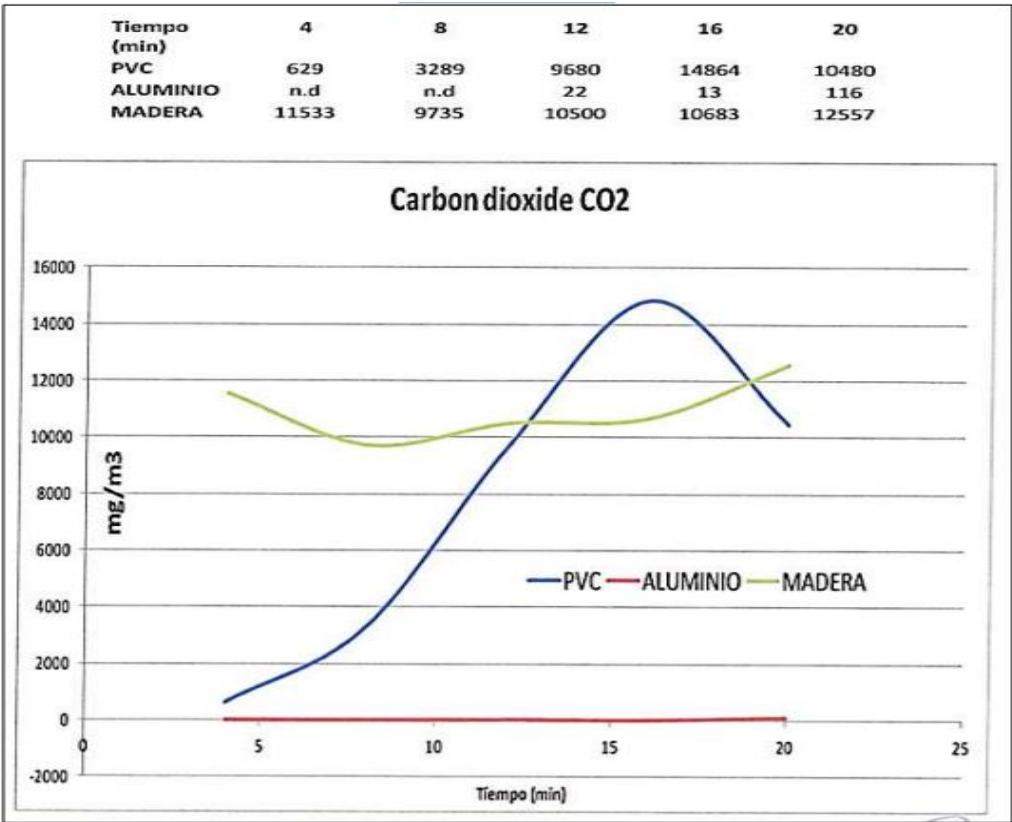
Fuente: Figura AC- 39: Emisiones de Dióxido de Carbono (CO 2 ) del aluminio según ensayo de toxicidad de gases. Adenda Complementaria.
