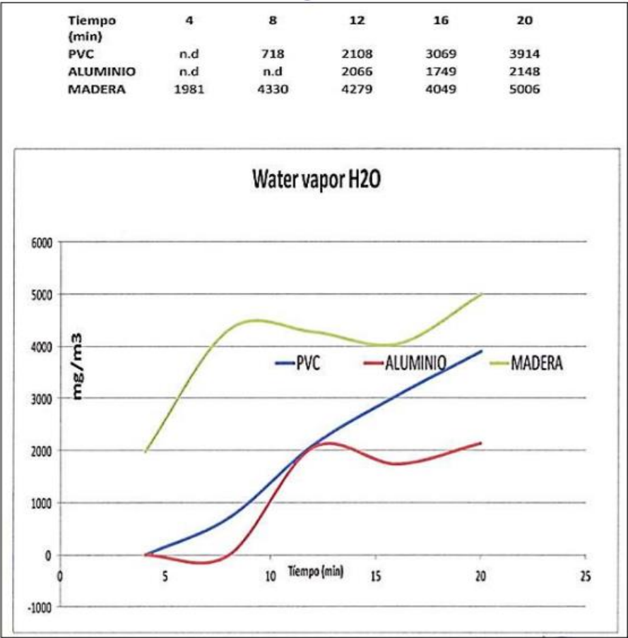
Fuente: Figura AC-37: Emisiones de Vapor de agua (H 2 O) del aluminio según ensayo de toxicidad de gases, Adenda Complementaria.
