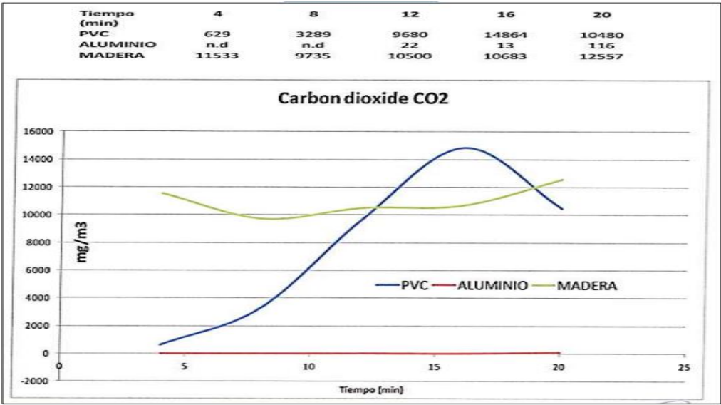
Fuente: Figura AC- 39: Emisiones de Dióxido de Carbono (CO2) del aluminio según ensayo de toxicidad de gases. Adenda Complementaria.
