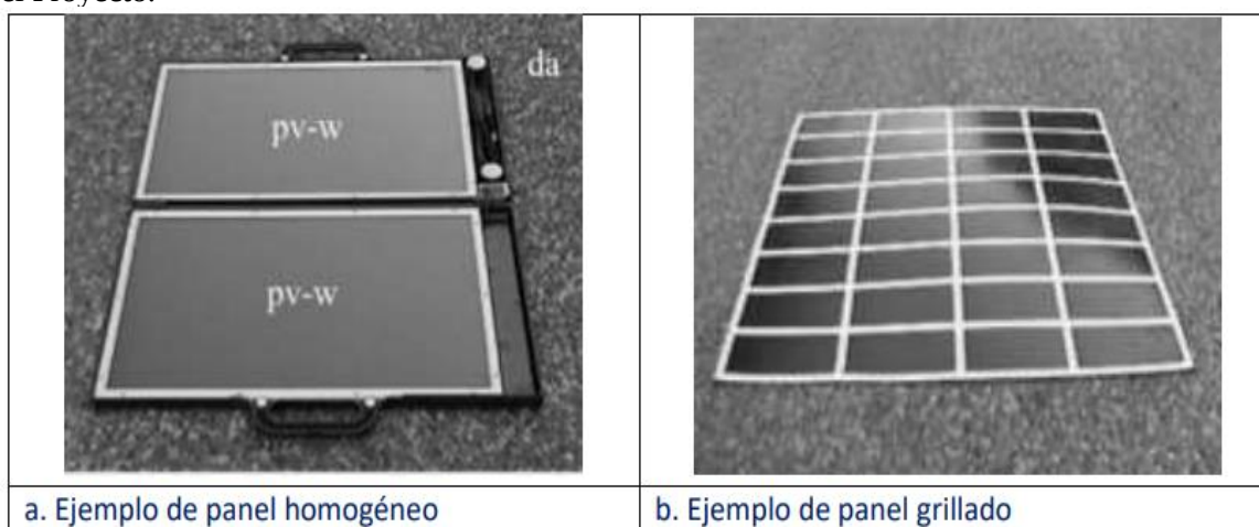
Figura: Comparación de Paneles Solares Homogéneos y Grillados y los que se usarán en el Proyecto.
