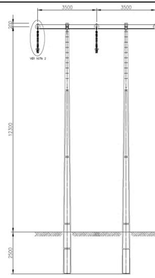
Figura 4-9 de la DIA, Estructura de anclaje – remate para transición entre el tramo aéreo y soterrado de la Línea 66 kV
