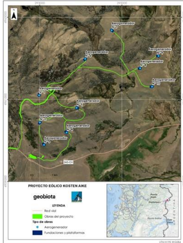
Figura 4-6 de la DIA Ubicación de Plataformas y Fundaciones para Aerogeneradores
