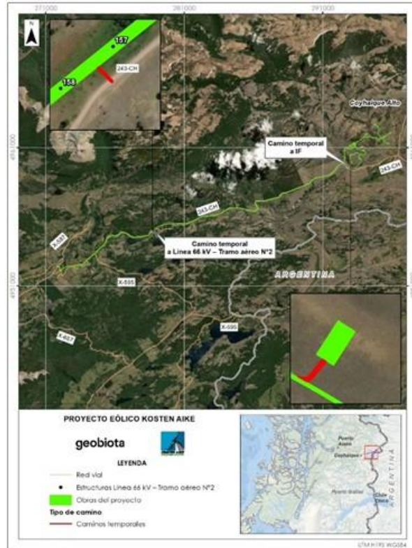
Figura 4-2. De la DIA “Caminos permanentes en Parque Eólico y S/E Las Bandurrias”
