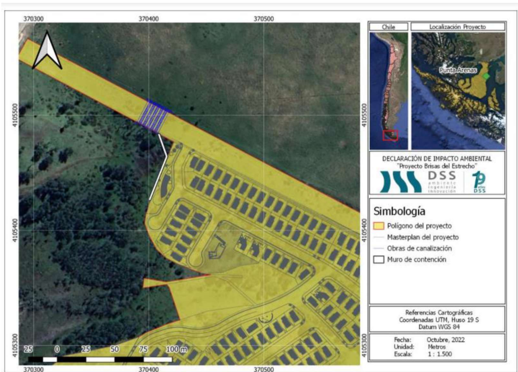
Figura 35. Planta de obras de canalización y muro de contención.
