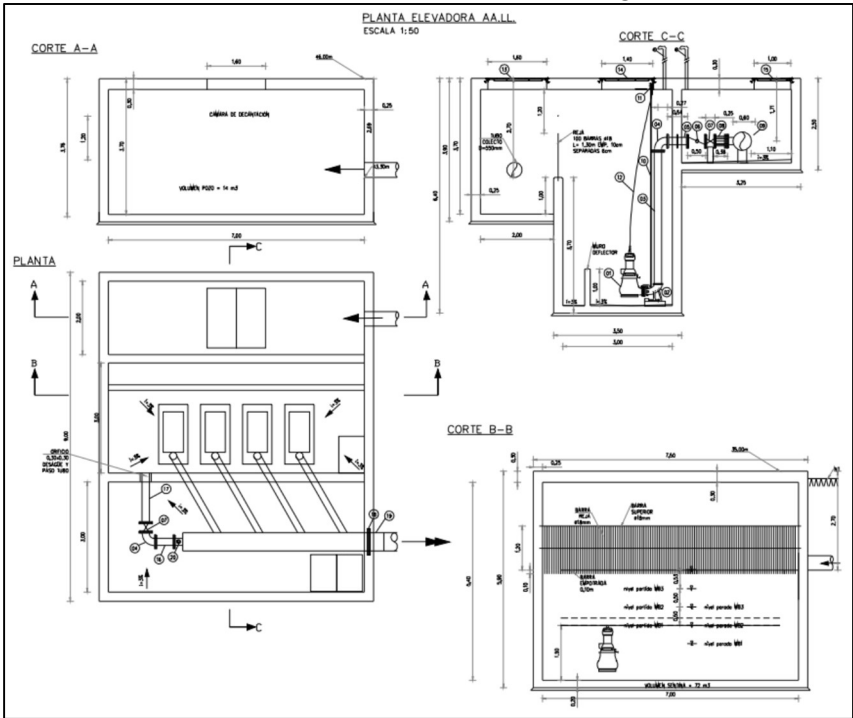
Figura 1. Boceto Planta Elevadora de Aguas Lluvias
