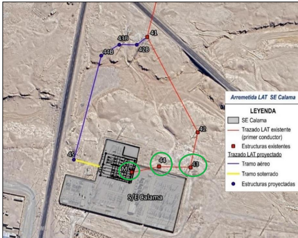
Imagen N°1: Estructuras existentes.
