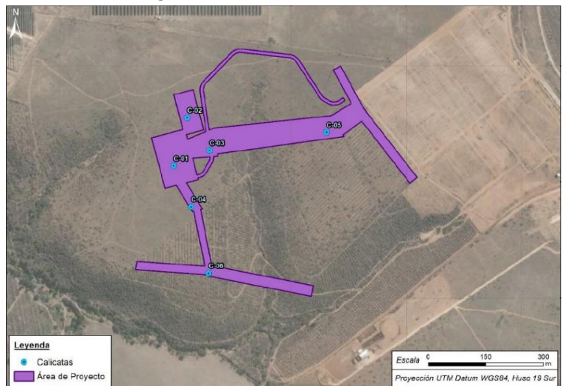
Figura 6.2.2 Ubicación de calicatas.
