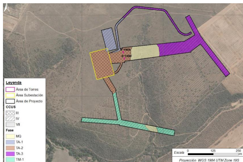
Figura 6.2.1. Área de afectación a unidad TA-2 CCUS III, sector subestación y estructuras N°139C y N°140A del Seccionamiento 220 kV.
