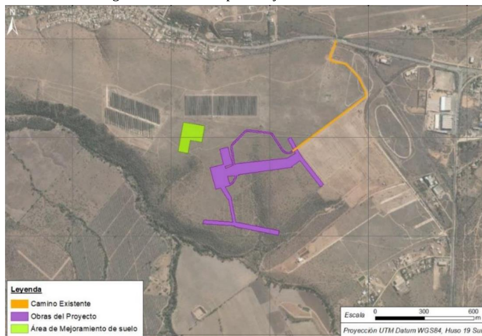
Figura 11.1.4.1 Área plan mejoramiento de suelo.
