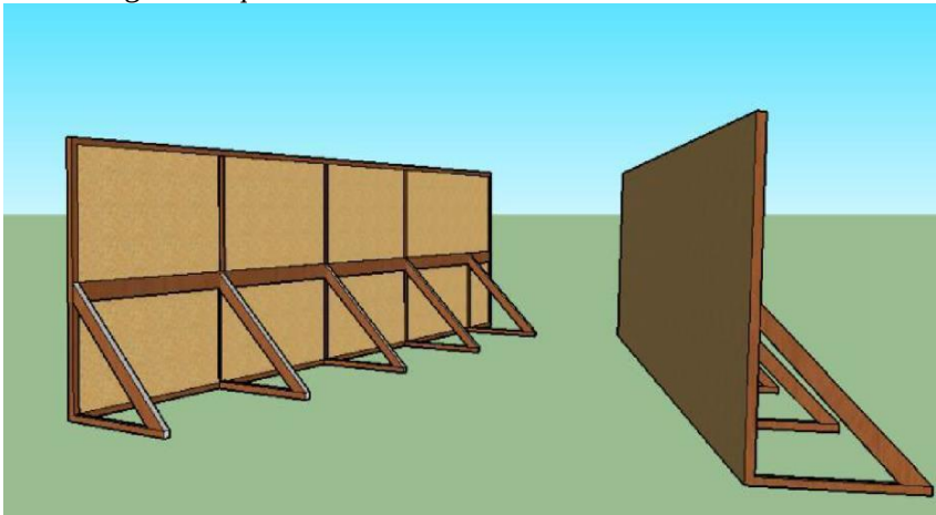
Figura: Esquema de barrera acústica modular trasladable.
