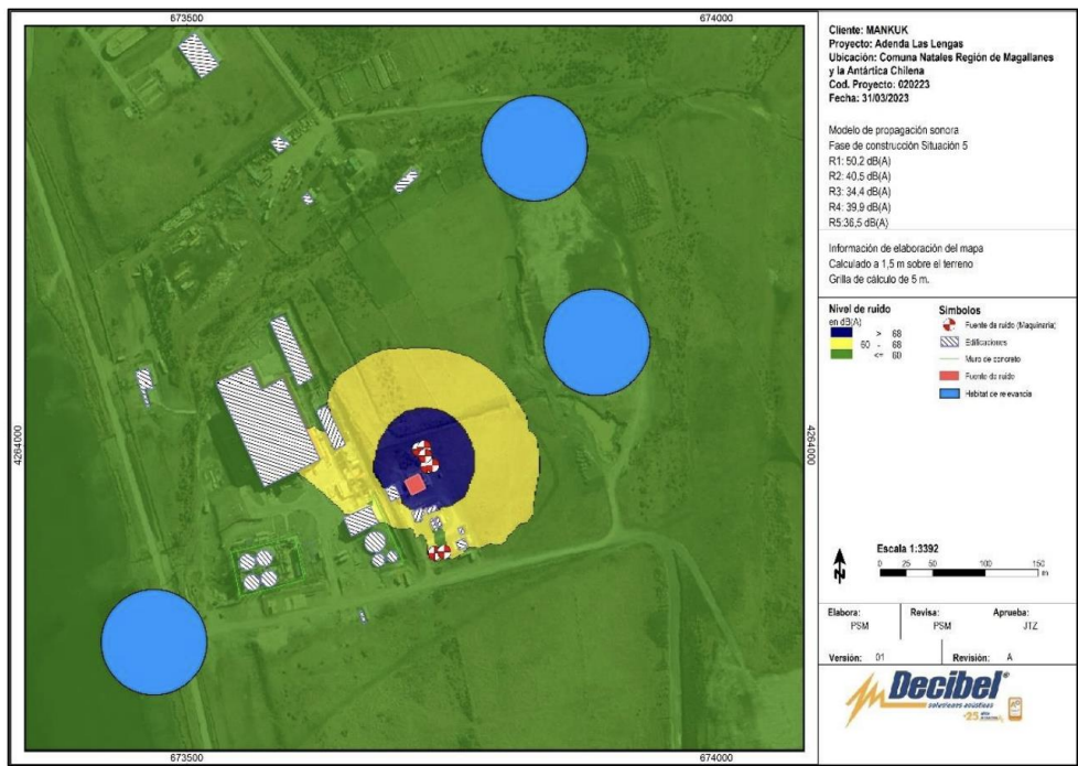
Figura 4 Proyección de fuentes de ruido para avifauna en fase de construcción. Fuente: ESTUDIO ACÚSTICO PARA DECLARACIÓN DE IMPACTO AMBIENTAL (Adenda)
