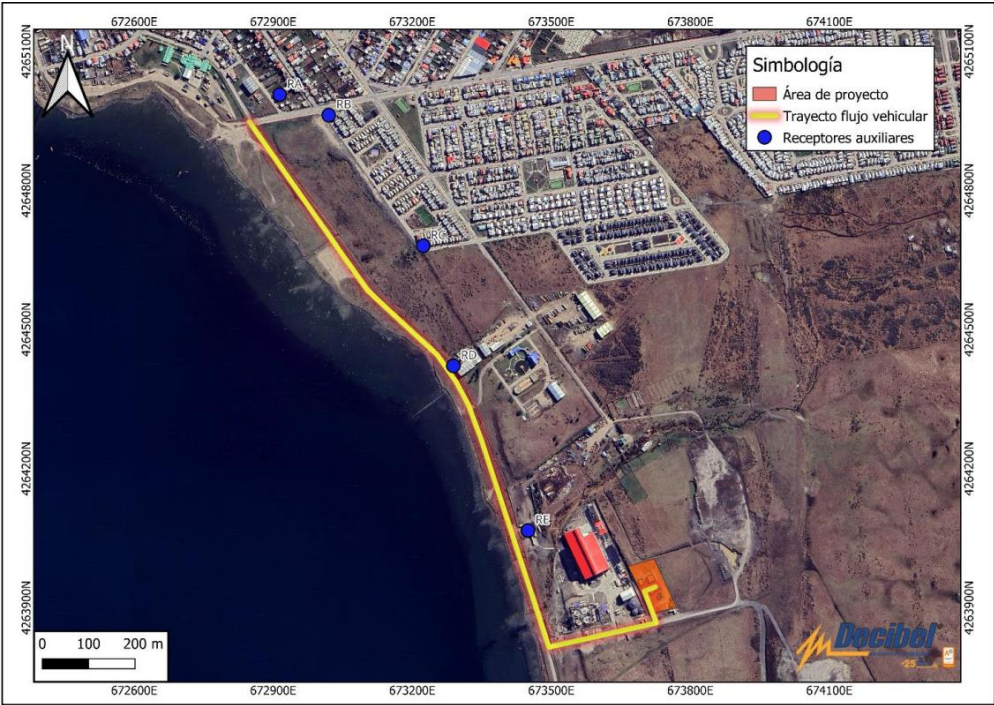
Figura 1 : Trayecto de flujo vehicular y receptores auxiliares al Estudio de Emisión de Ruido y Vibración. Fuente: ANEXO B: ESTUDIO ACÚSTICO Y VIBRACIONES (Adenda Complementaria)
