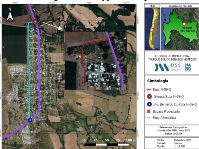
Figura 5.2.6. Bypass Tucapel
