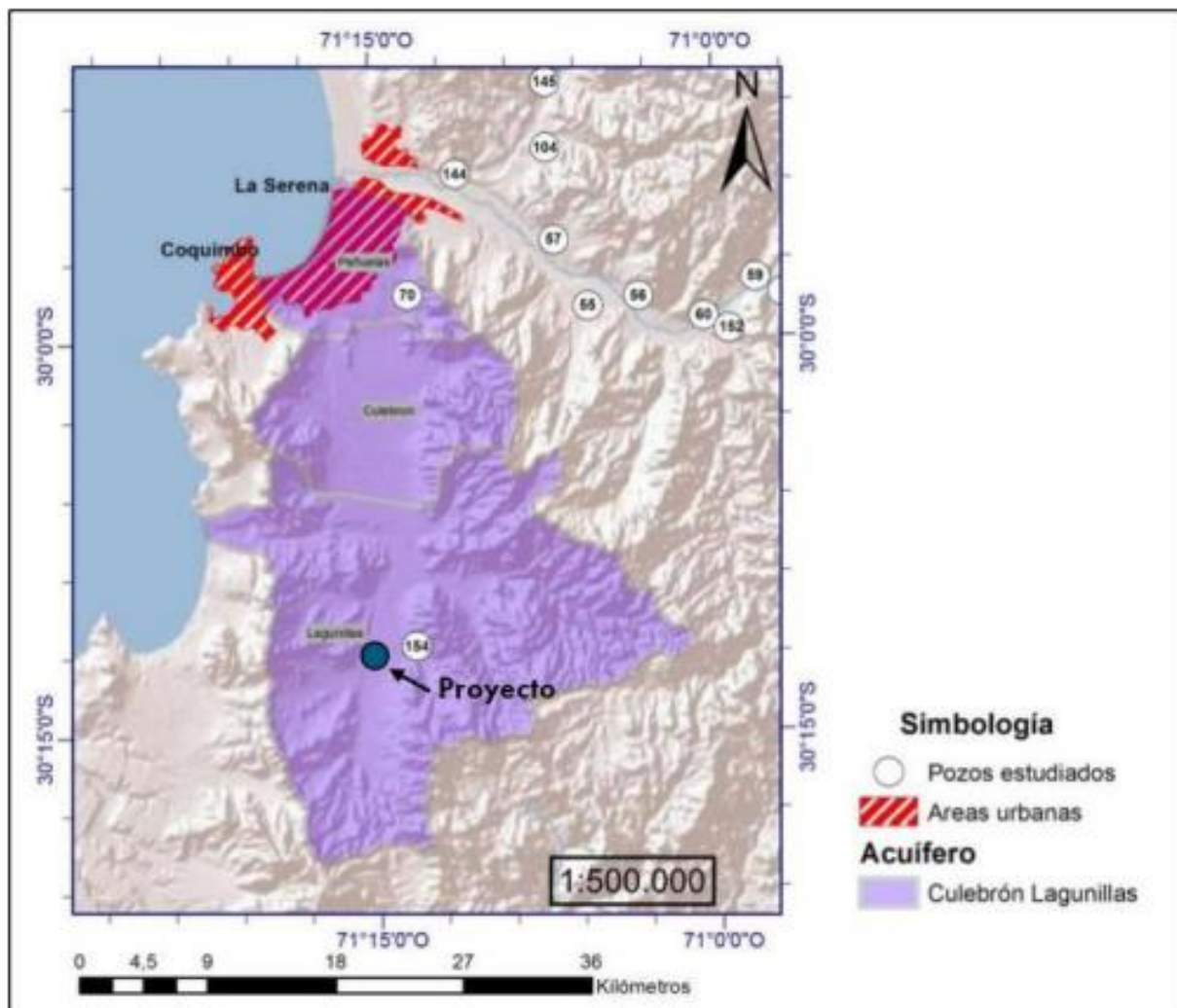
Figura 4. Al Hidrogeología.
