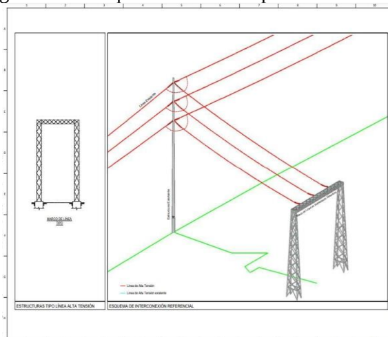
Figura 4.2.3. Esquema referencial punto de conexión.
