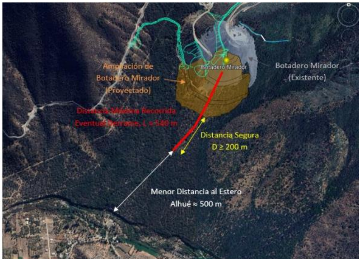
Figura 4: Distancia de viaje o recorrido del estéril derramado sin considerar el pretil de contención
