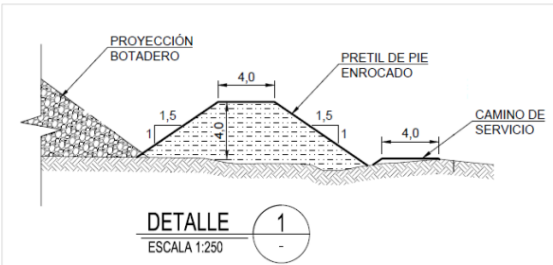
Figura 2: Sección del Pretil basal de contención del Botadero
