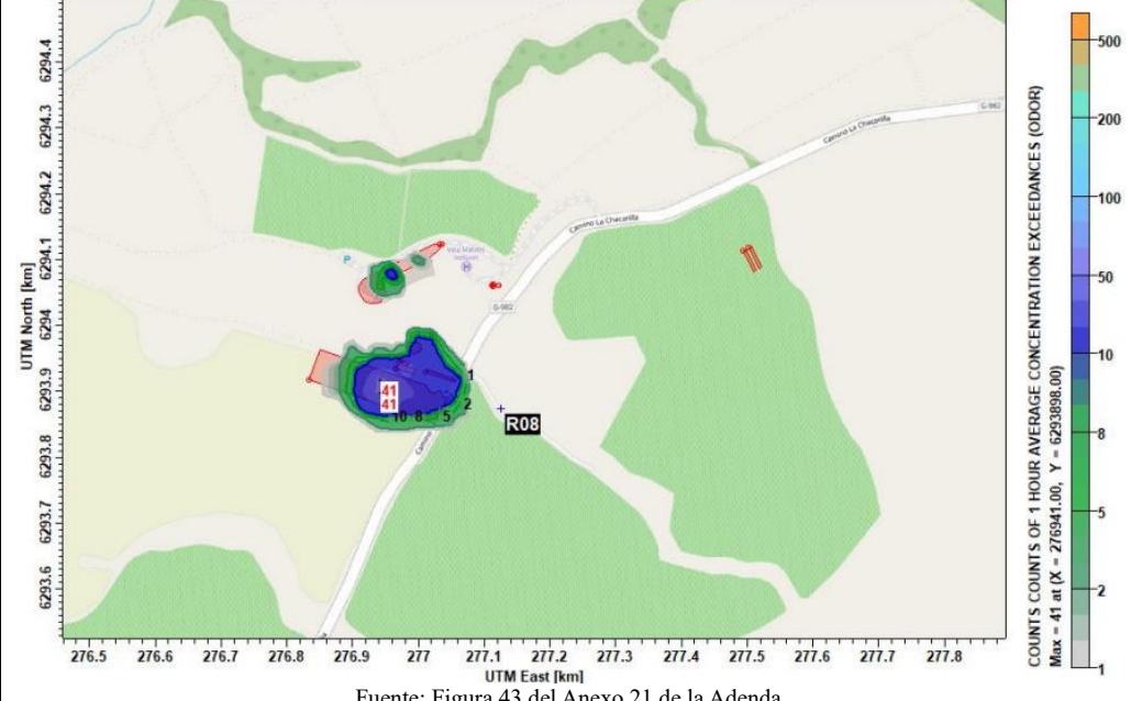
Figura 14: Isolínea de concentración de olor, hora de excedencia de 5 Uo.
