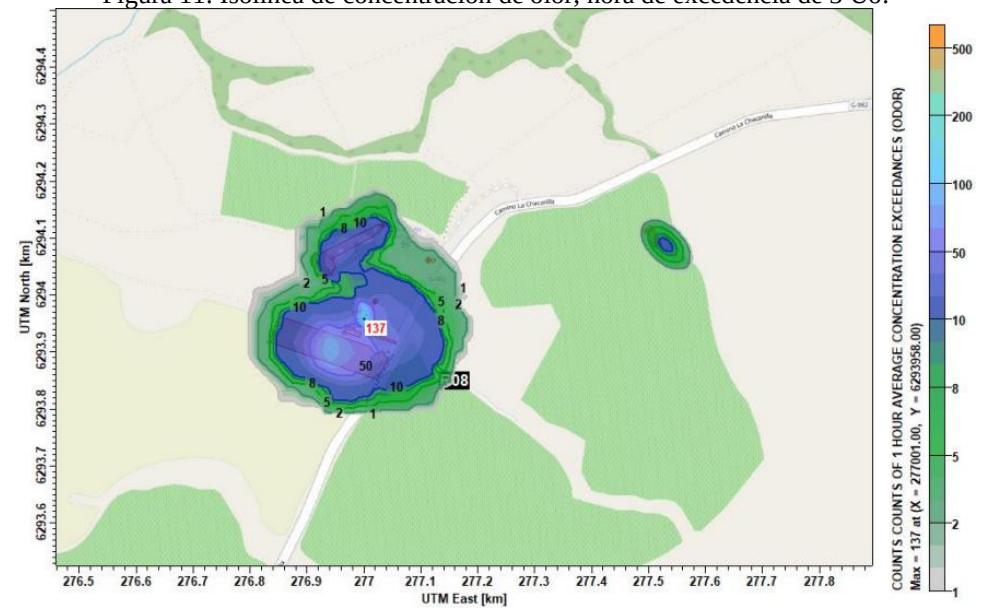
Figura 11: Isolínea de concentración de olor, hora de excedencia de 3 Uo.
