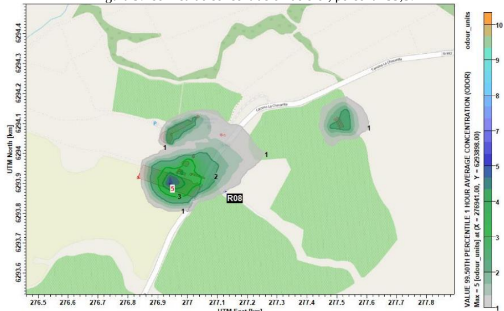
Figura 9: Isolínea de concentración de olor, percentil 99,5.
