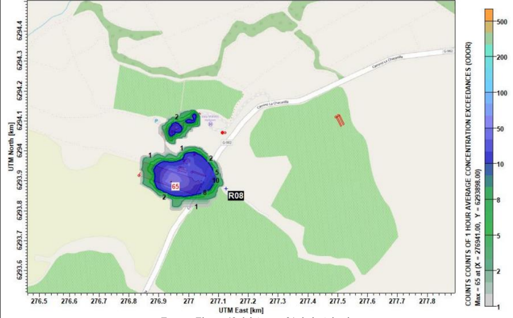
Figura 13: Isolínea de concentración de olor, hora de excedencia de 4 Uo.
