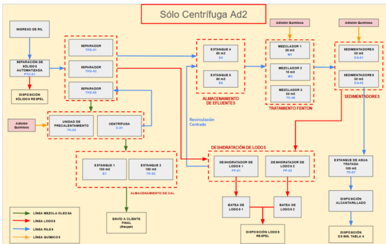
Figura 13.3: Diagrama de proceso - Fases Operativas 1 y 2.
