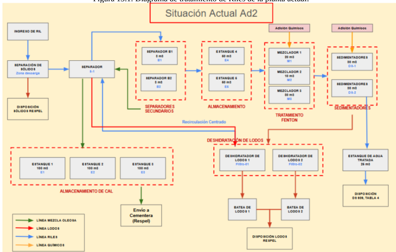
Figura 13.1: Diagrama de tratamiento de Riles de la planta actual.
