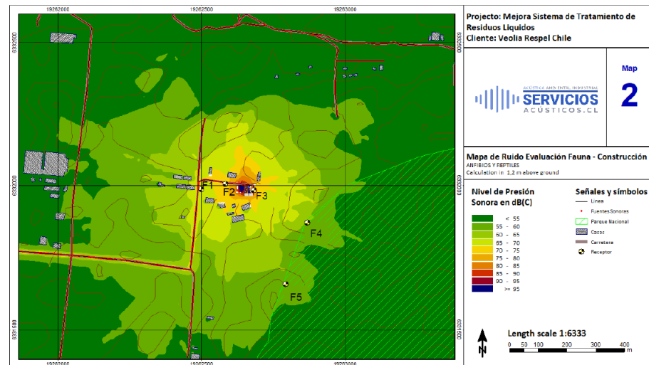
Figura 4.6.4.3.3: Modelo de Propagación Sonora en Evaluación Anfibios y Reptiles. Fase de Construcción.
