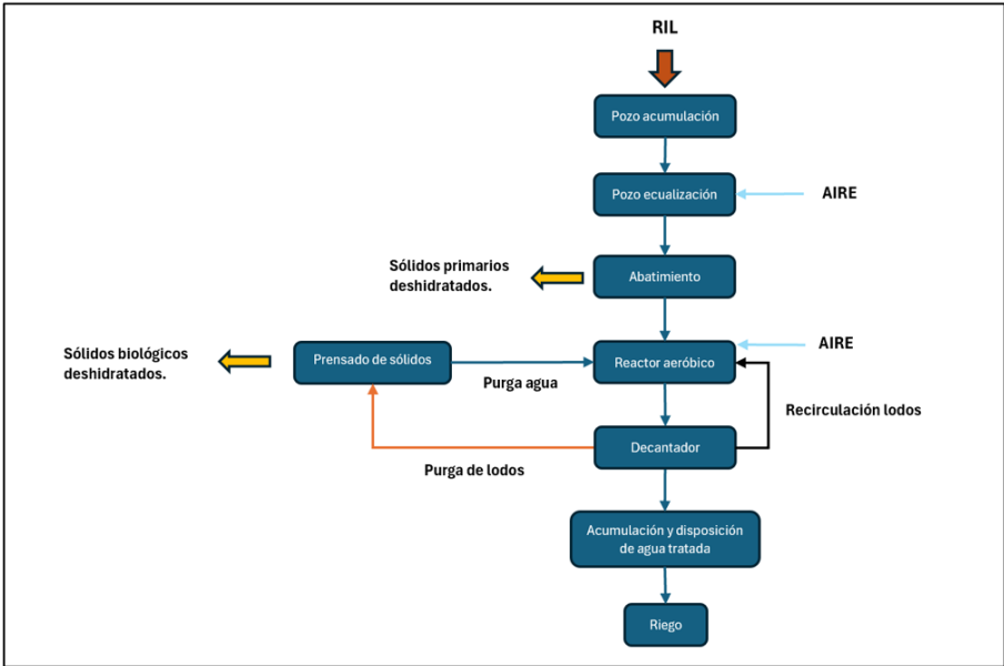
Figura 4.7.1.2.1: Diagrama proceso de depuración.
