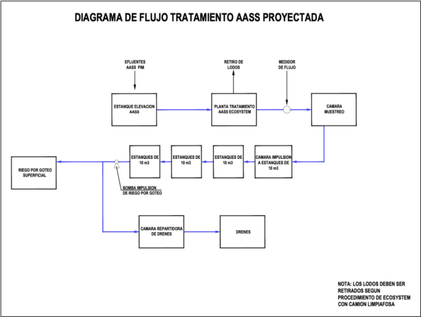
Fuente: Figura 1-13: Diagrama de flujo, aguas servidas, Capítulo Descripción de Proyecto Actualizado de la Adenda Complementaria.
