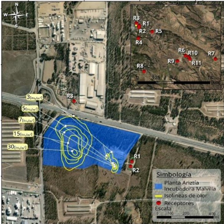
Figura 4.3.2.5 Curvas isodoras todas las fuentes – CP98-1hr=3 [ouE/m³] – E. Futuro.
