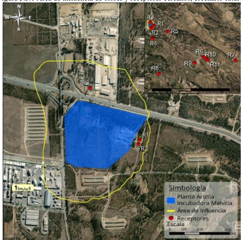
Figura 5.3.1 Área de influencia de olores y receptores cercanos, escenario futuro.
