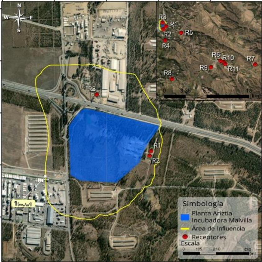
Figura 4.3.2.4 Área de influencia 1 [ouE/m³] – E. Futuro.
