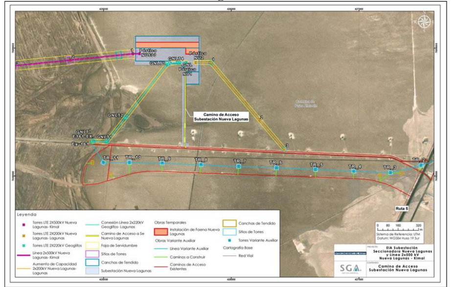
Figura N°4.1.2. Camino de acceso a Subestación seccionadora Nueva Lagunas
