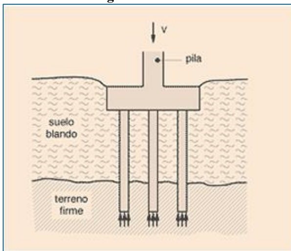
Figura N°4.6.1.2.3: Imagen referencial fundación Micropilote
