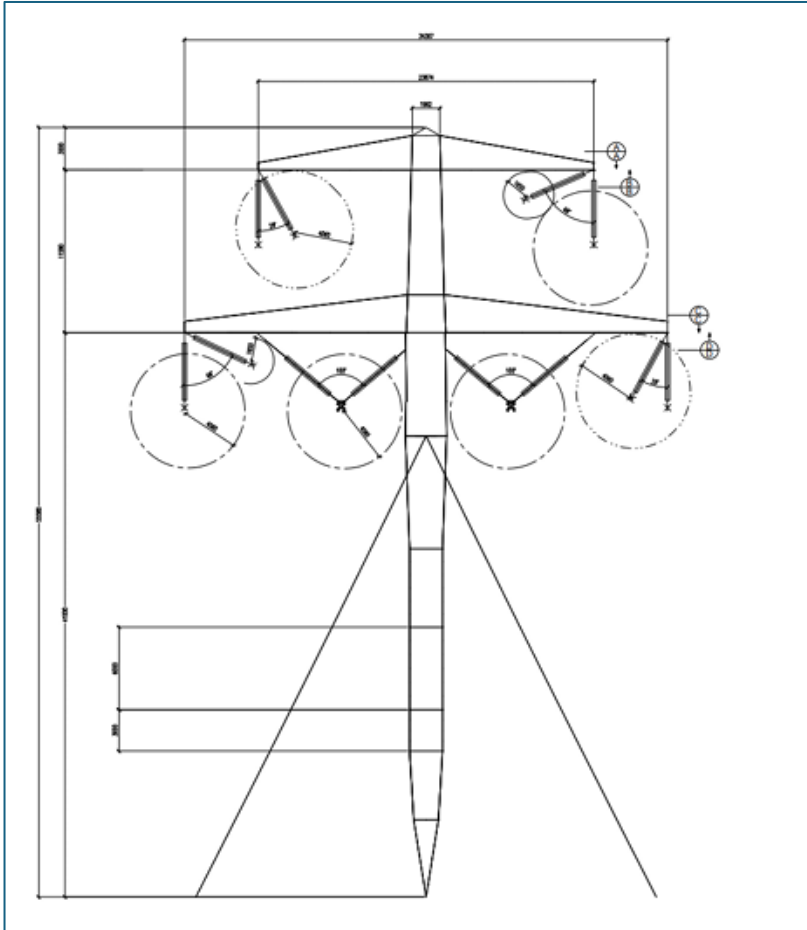
Figura N°4.6.1.2.5: Estructura atirantada LAT 2x500 kV
