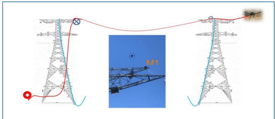
Figura N°4.6.1.2.5: Imagen referencial de tendido de conductor por dron
