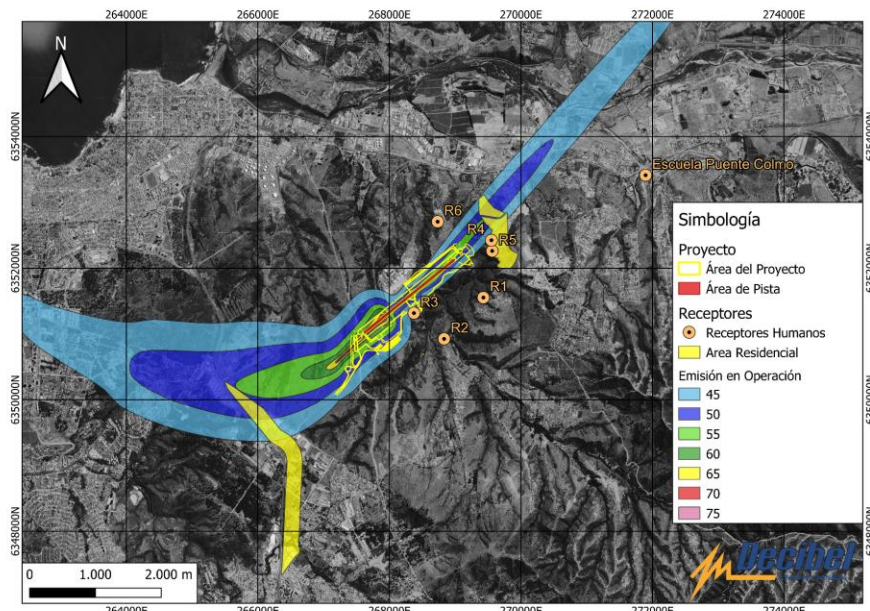
Figura 4.7.5.3.1: Mapa de ruido en fase de operación, contornos YDNL.
