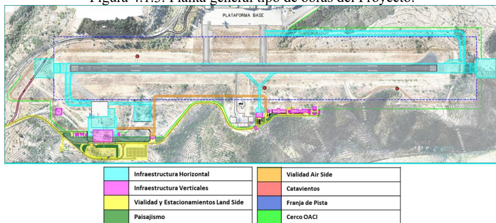
Figura 4.1.3: Planta general tipo de obras del Proyecto.
