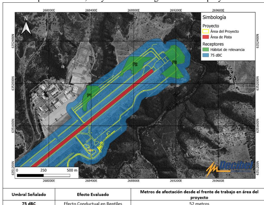
Figura 4.6.4.3.4: Mapa de ruido en fase de construcción, frente de trabajo para reptiles en dBC, Proyección a lo largo del área del proyecto.
