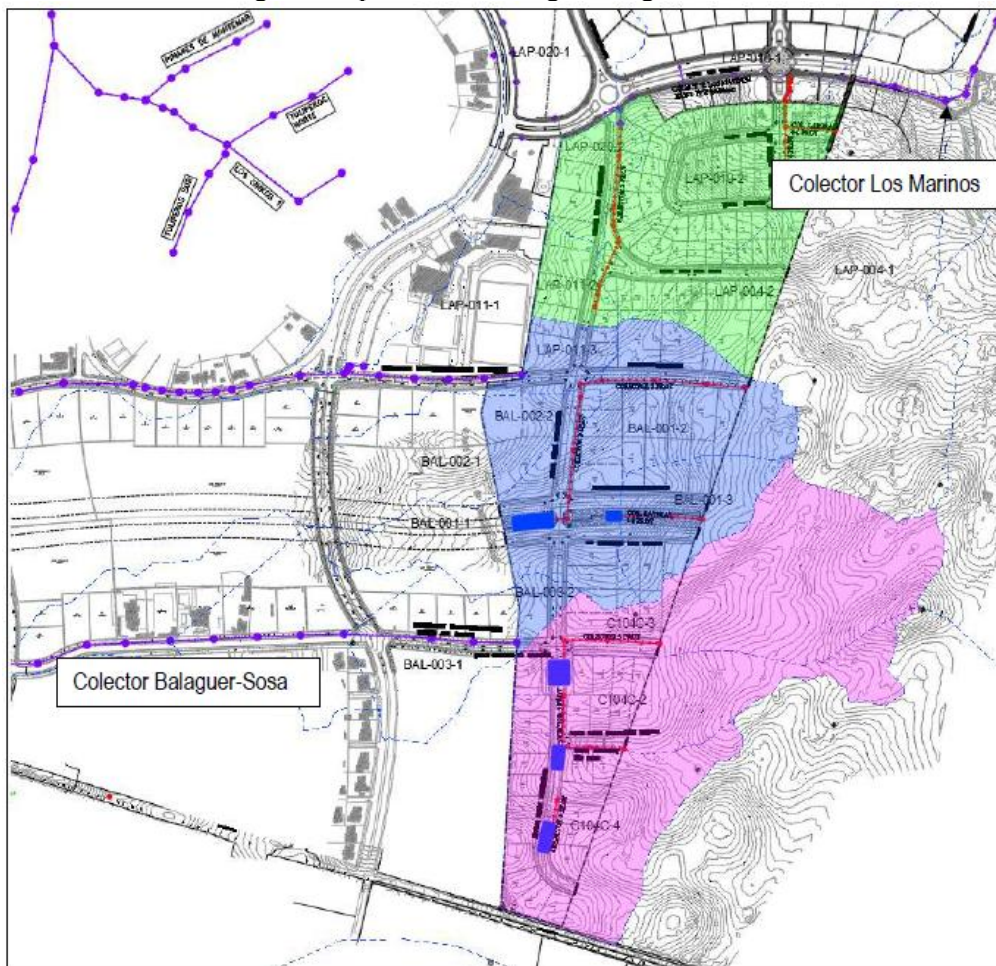
Figura: Esquema de descargas de aguas lluvias.
