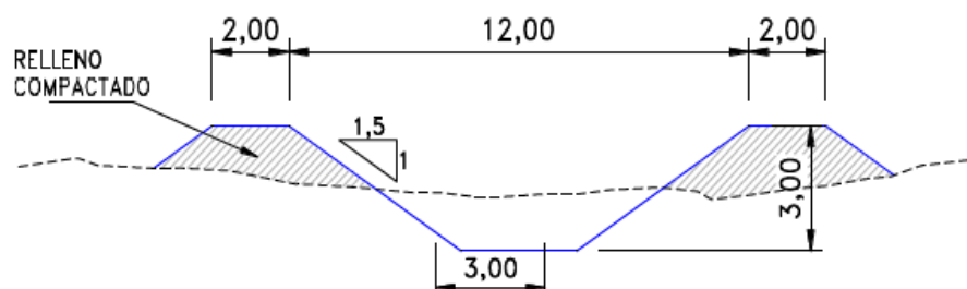
Fuente: Figura 4 del Anexo 16 de la Adenda Complementaria de la DIA. Sección Tipo.
