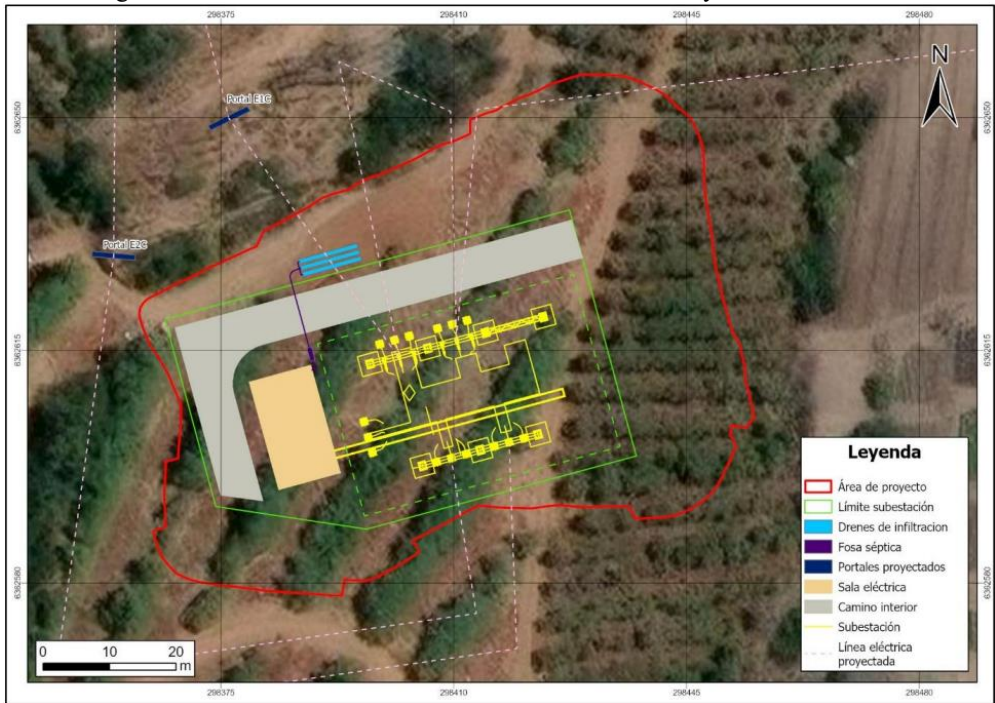
Figura 4.2.3: Obras Permanentes – Subestación eléctrica y seccionamientos.
