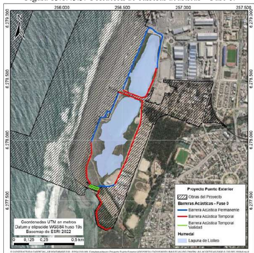
Figura 13.1.43.3: Ubicación de barreras acústicas – Fase 0.
