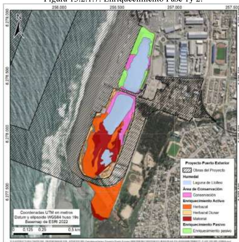
Figura 13.2.1.7: Enriquecimiento Fase 1y 2.
