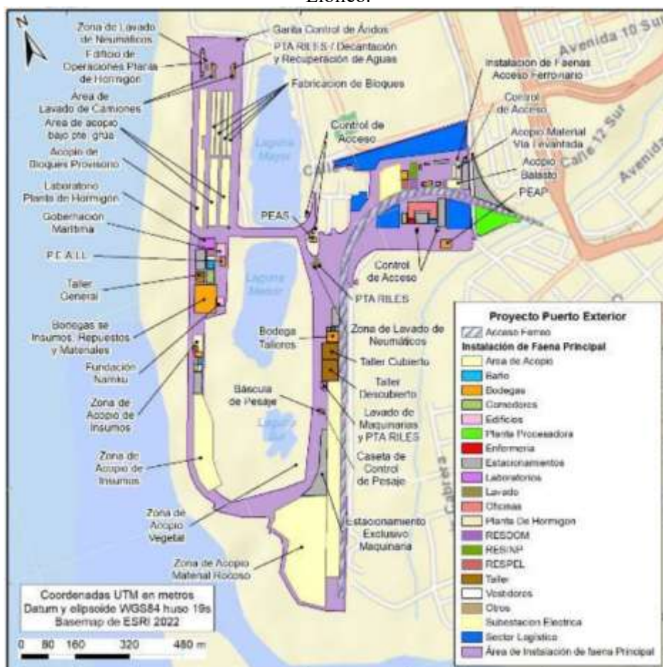
Figura 6.1.3.2: Localización de partes y obras alrededor de las Lagunas de Lollole.
