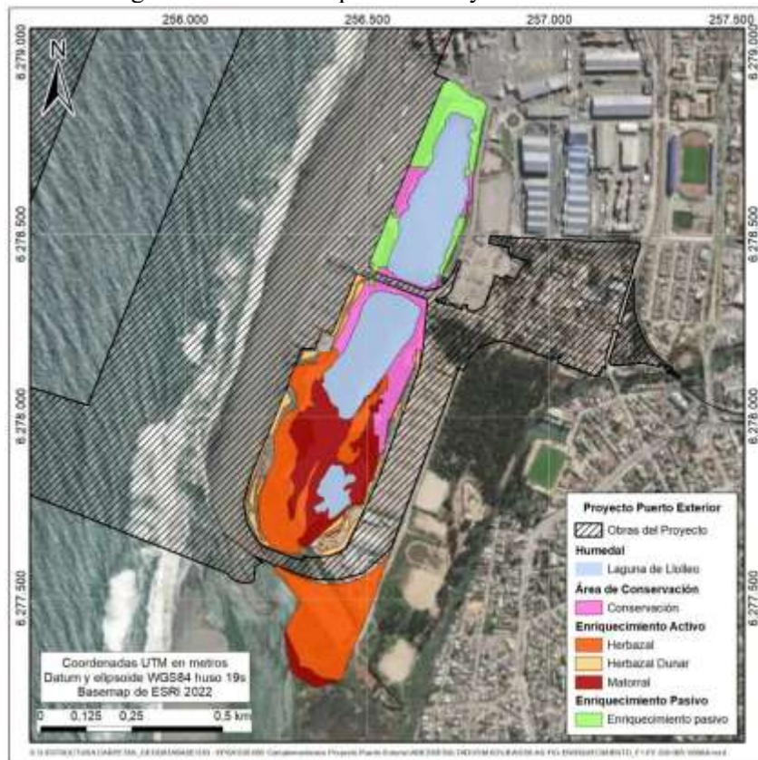
Figura 13.2.1.2: Enriquecimiento y renaturalización.
