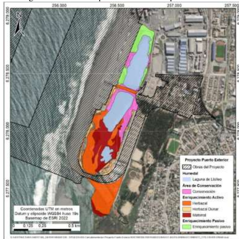
Figura 13.2.1.9: Enriquecimiento. Fase Operación Plena.
