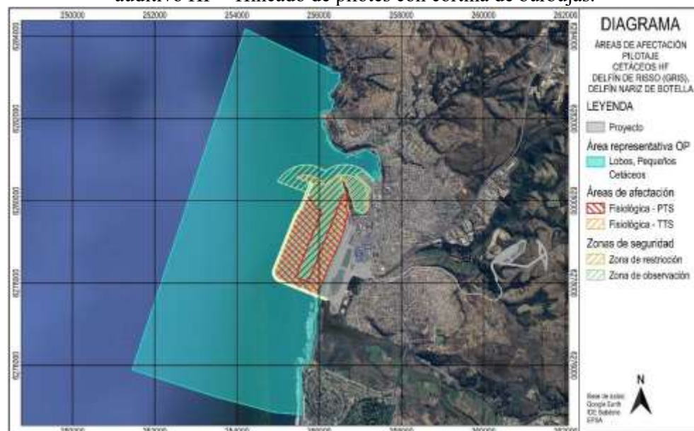
Figura 13.1.25.10: Áreas de efectos fisiológicos y Zonas de seguridad – Grupo auditivo HF – Hincado de pilotes con cortina de burbujas.
