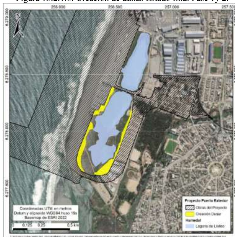
Figura 13.2.1.6: Creación de dunas Estado final Fase 1y 2.
