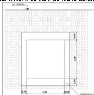
Figura 8.3.2: Diseño de paso de fauna durante la Fase 0.
