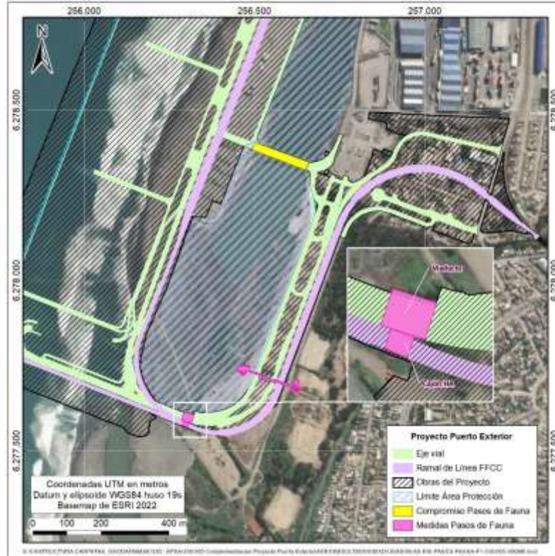
Figura 13.1.8.2: Resumen de los pasos de fauna en Fase 1, 2 y Operación plena.
