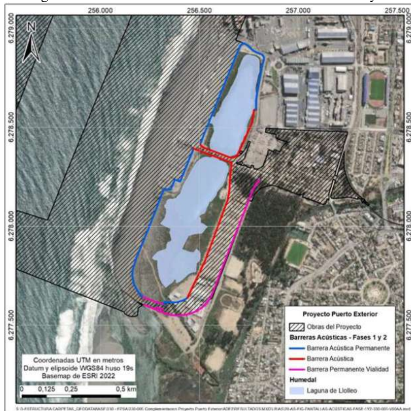
Figura 13.1.43.2: Ubicación de barreras acústicas – Fase 1 y 2.
