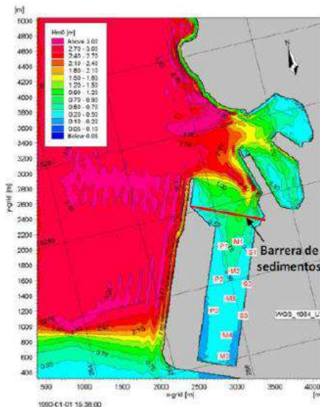
Figura 8.4.2: Ubicación de cortinas de burbujas.
