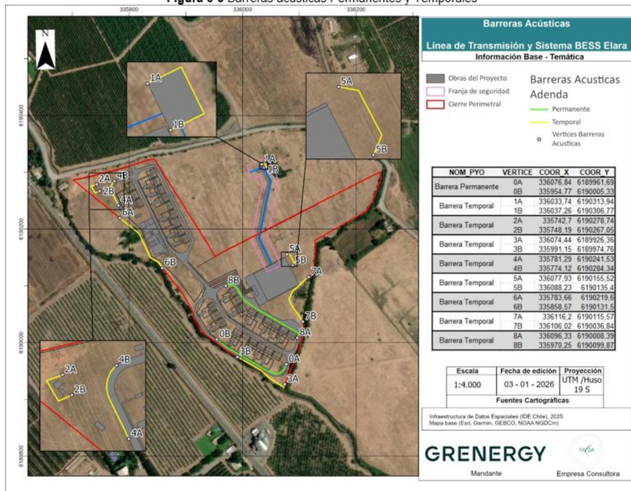
Figura 6-3 Barreras acústicas Permanentes y Temporales
