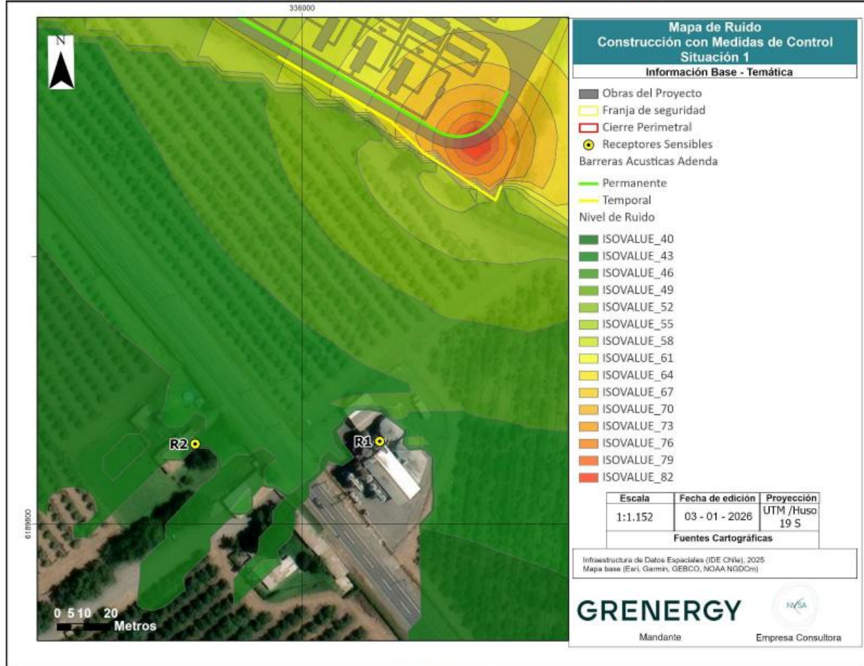
Figura 6-5 Mapa de Ruido Construcción con Acciones de Control S1
