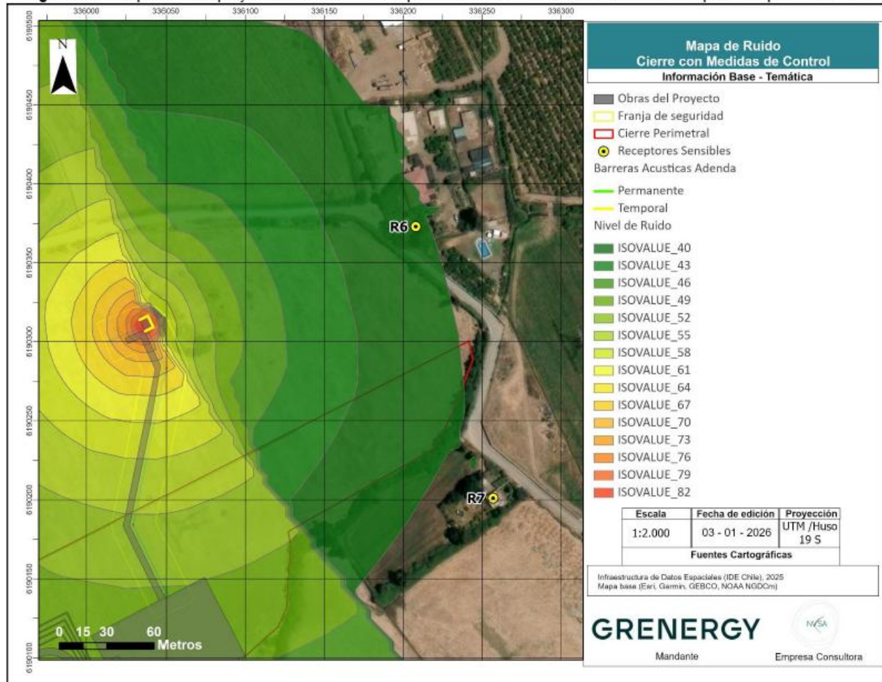
Figura 6-15: Mapa de ruido proyectado en SoundPLAN para fase de cierre con acciones de control para receptores R6 – R7.
