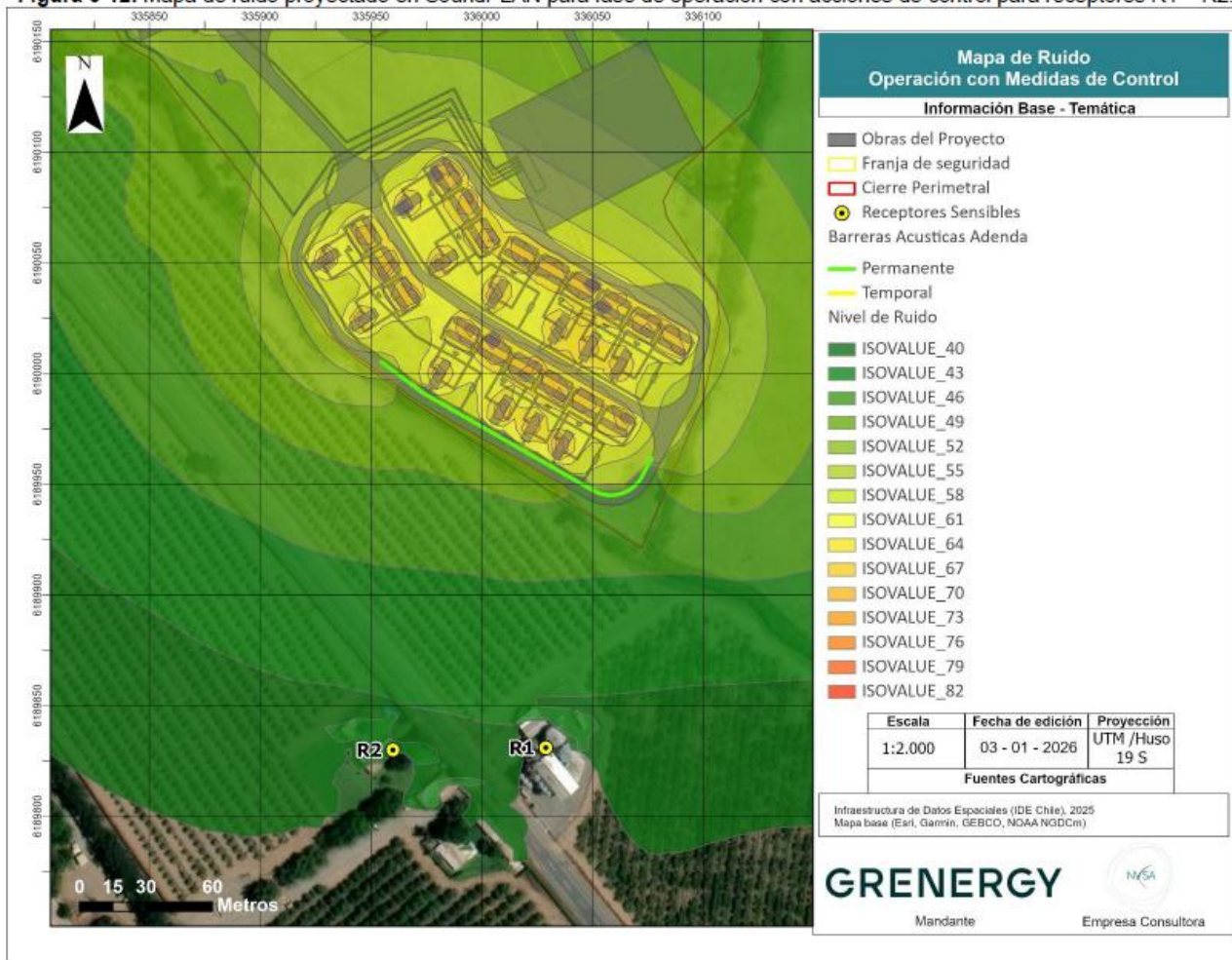
Figura 6-12: Mapa de ruido proyectado en SoundPLAN para fase de operación con acciones de control para receptores R1 – R2.
