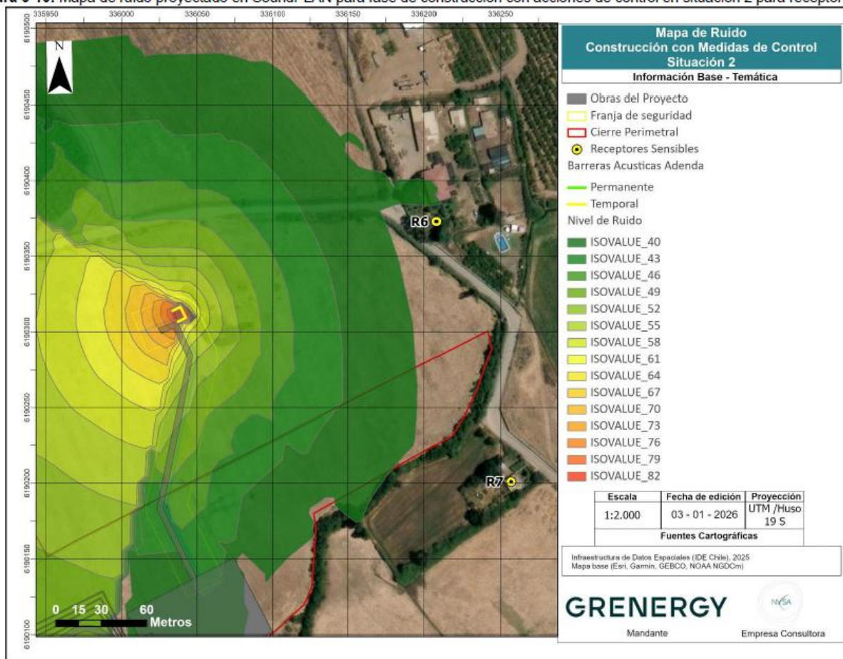
Figura 6-10: Mapa de ruido proyectado en SoundPLAN para fase de construcción con acciones de control en situación 2 para receptores R6.
