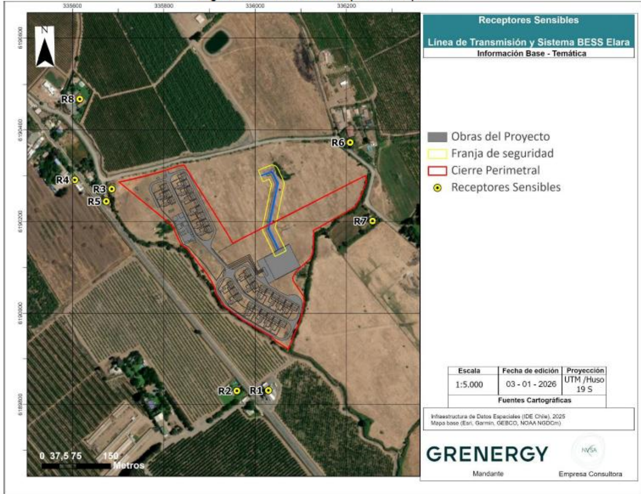
Figura 3-2: Identificación de puntos receptores.
