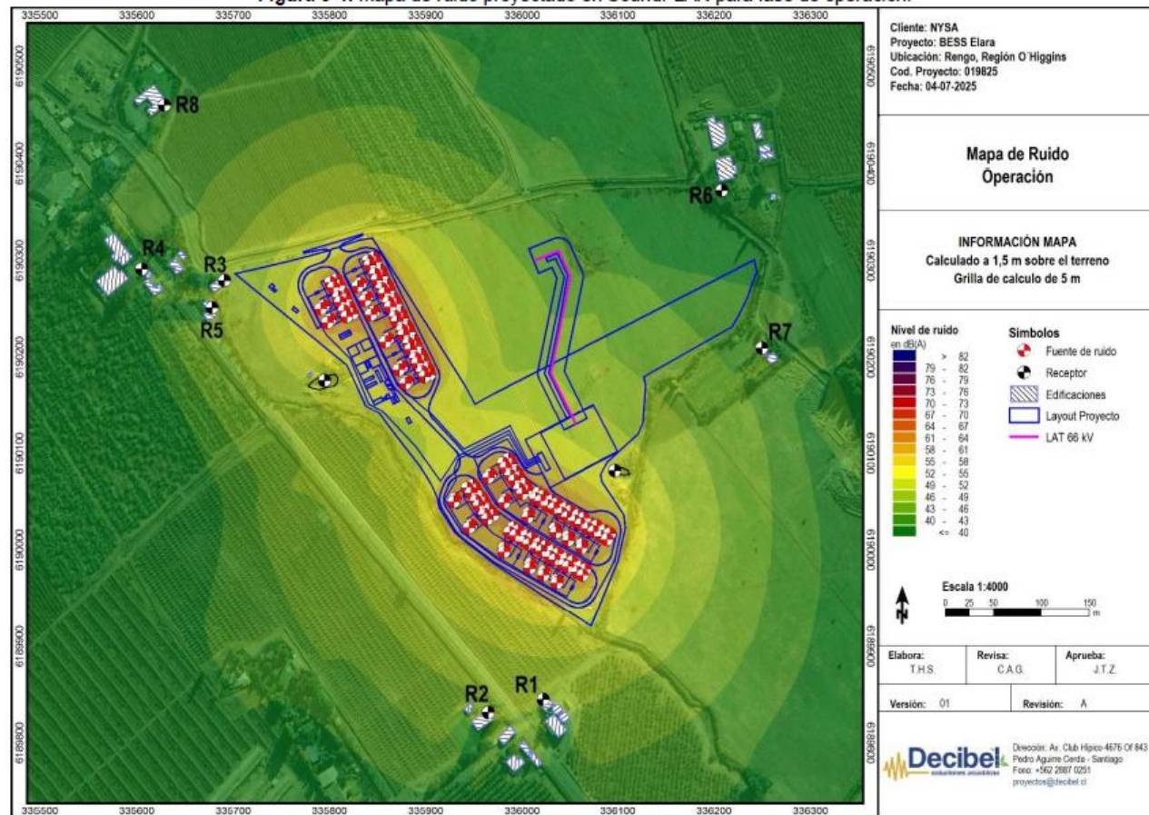
Figura 5-4: Mapa de ruido proyectado en SoundPLAN para fase de operación.
