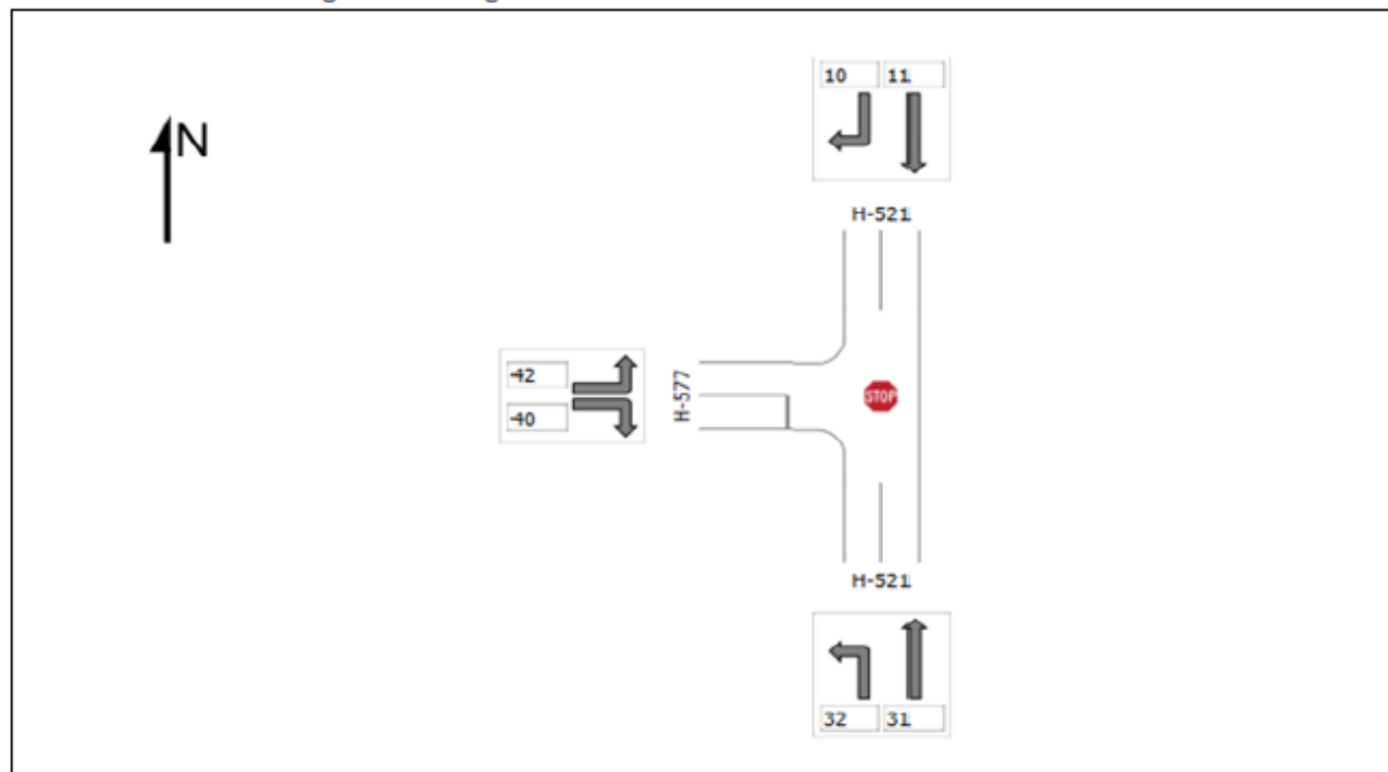
Figura 15. Diagrama intersección N°2 Ruta H-521 con H-577
