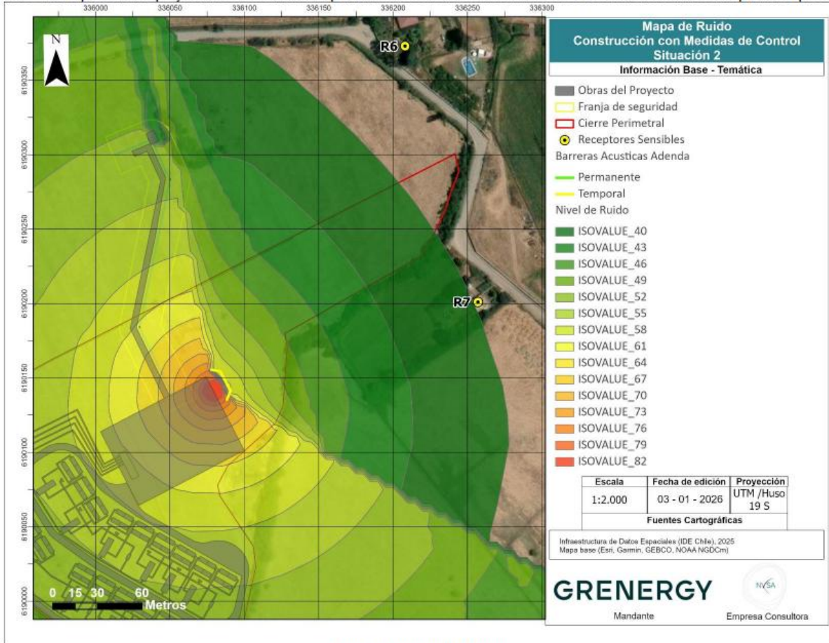
Figura 6-11: Mapa de ruido proyectado en SoundPLAN para fase de construcción con acciones de control en situación 2 para receptores R7.
