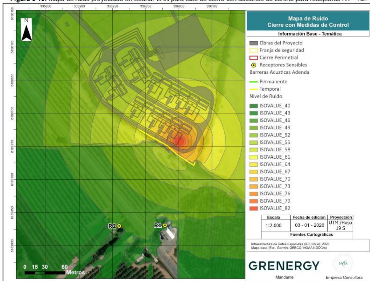
Figura 6-13: Mapa de ruido proyectado en SoundPLAN para fase de cierre con acciones de control para receptores R1 – R2.
