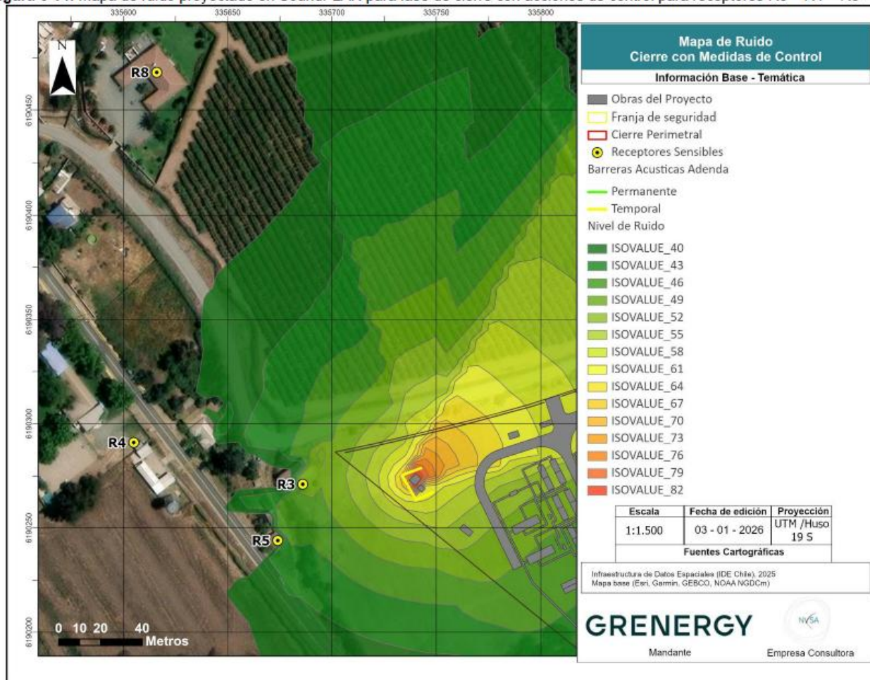
Figura 6-14: Mapa de ruido proyectado en SoundPLAN para fase de cierre con acciones de control para receptores R3 – R4 – R5 – R8
