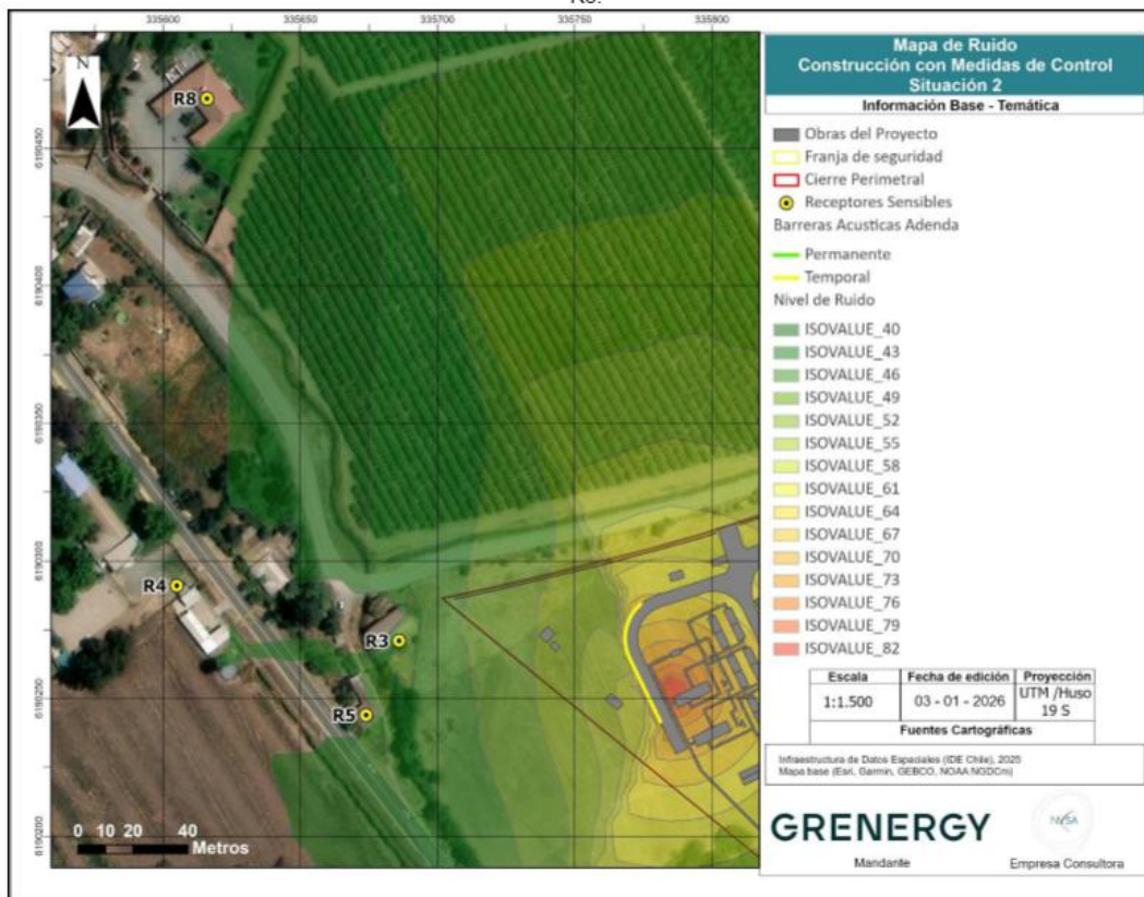
Figura 6-9: Mapa de ruido proyectado en SoundPLAN para fase de construcción con acciones de control en situación 2 para receptores R3 – R4 – R5 – R8.
