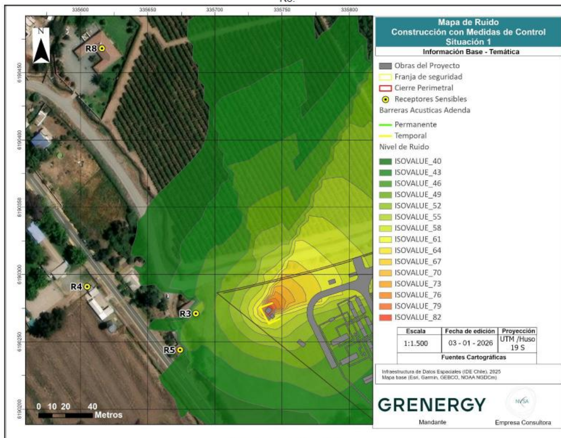
Figura 6-6: Mapa de ruido proyectado en SoundPLAN para fase de construcción con acciones de control en situación 1 para receptores R3 – R4 R8.
