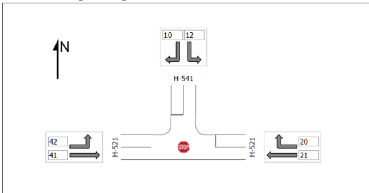
Figura 16. Diagrama intersección N°3: Ruta H-521 con H-541
