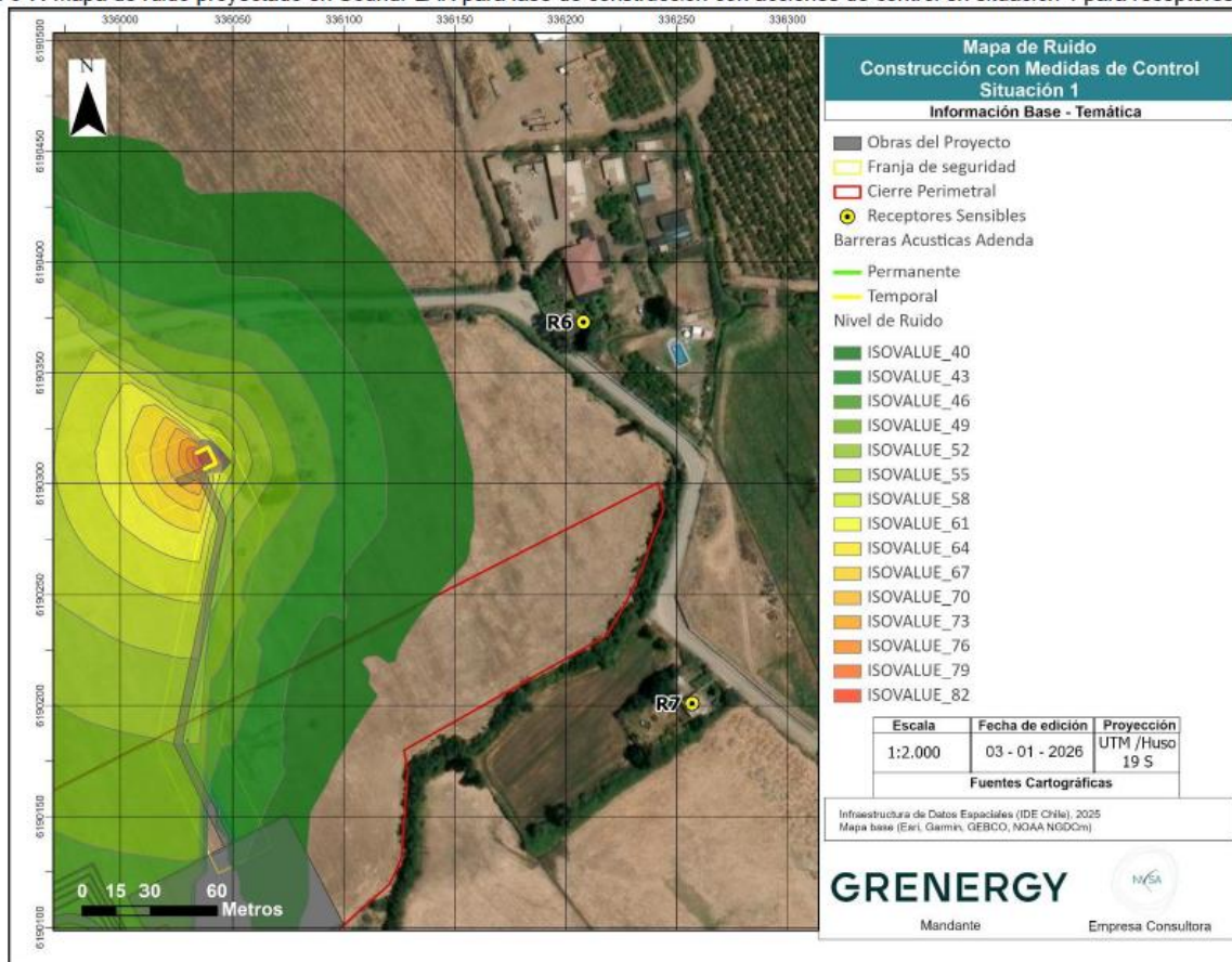
Figura 6-7: Mapa de ruido proyectado en SoundPLAN para fase de construcción con acciones de control en situación 1 para receptores R6 – R7.
