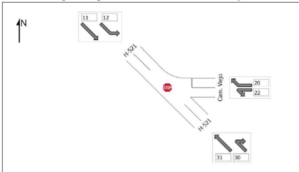
Figura 14. Diagrama intersección N°1 Ruta H-521 con Cam. Viejo
