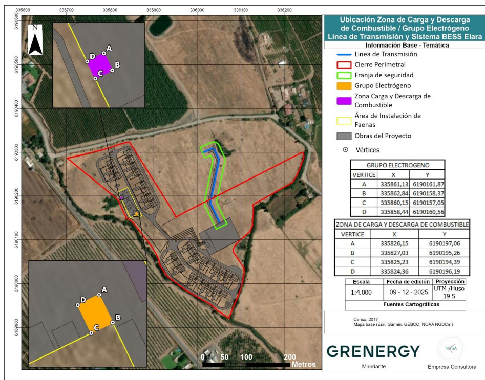
Fuente: Figura 1-1. Grupos electrógenos y zona de carga y descarga de combustible, de la Adenda (Parte A3).
