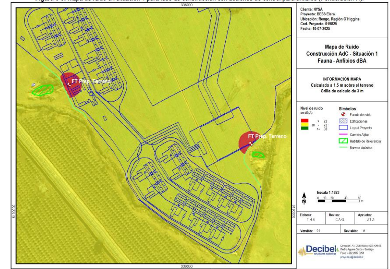
Figura 6-5: Mapa de ruido en situación 1 para fase de construcción con acciones de control para anfibios (Ponderación A).
