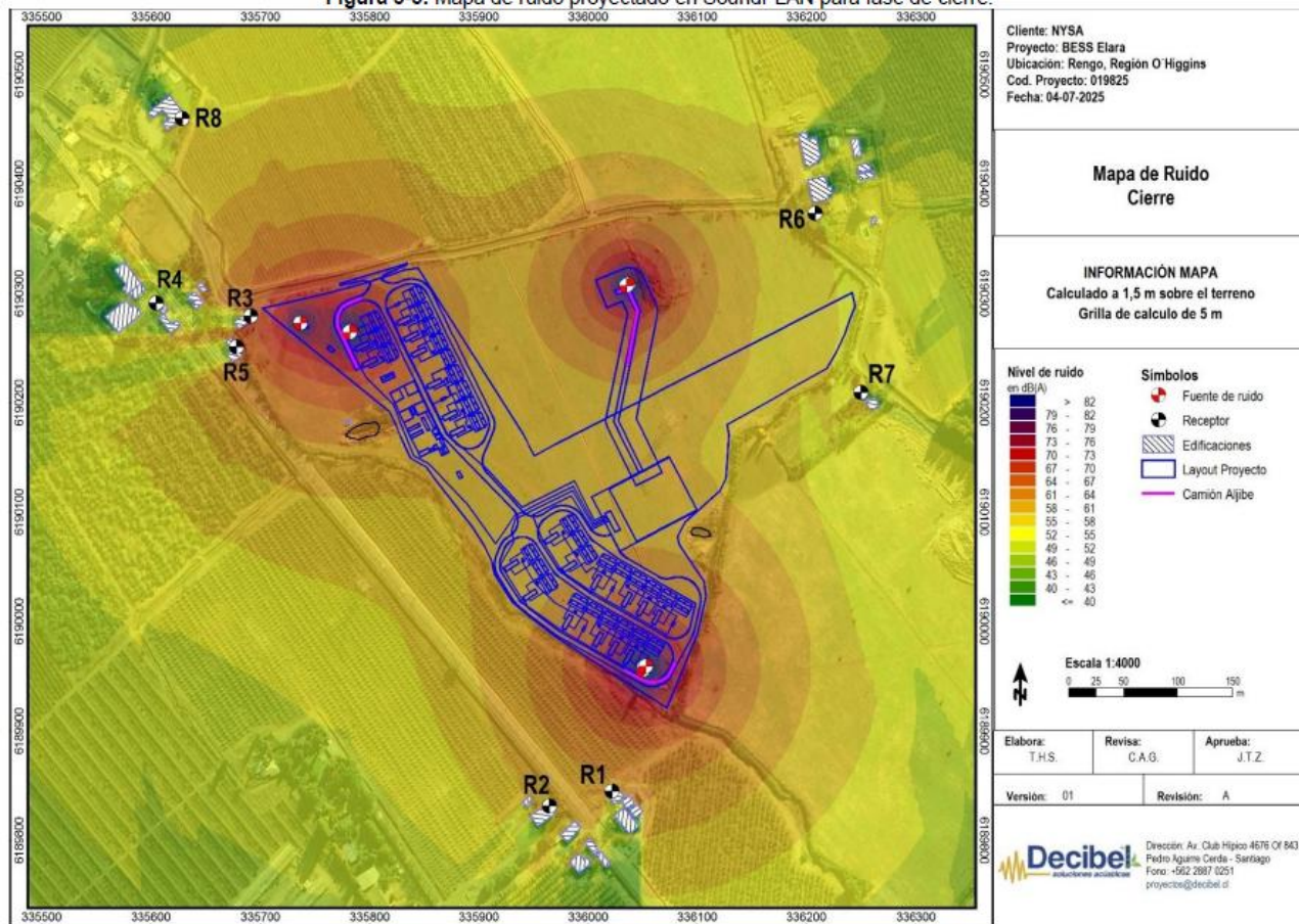
Figura 5-5: Mapa de ruido proyectado en SoundPLAN para fase de cierre.
