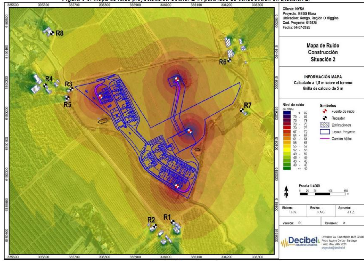
Figura 5-3: Mapa de ruido proyectado en SoundPLAN para fase de construcción en situación 2.
