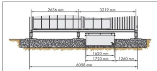
Figura 1-14. Posición de Contenedor Anti-Derrame de Aceite
