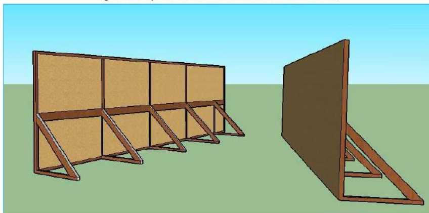
Figura 24: Esquema de barrera acústica modular trasladable,
