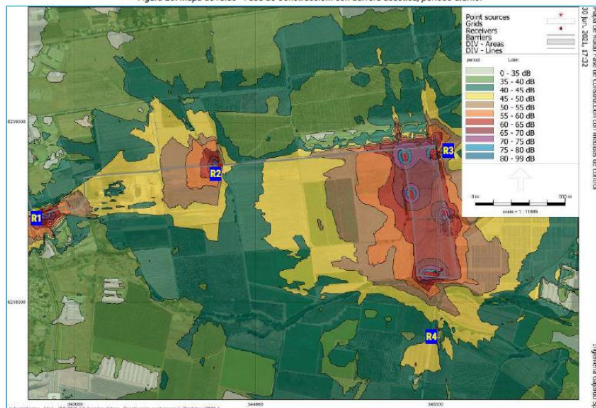
Figura 28: Mapa de ruido - Fase de Construcción: con barrera acústica, periodo diurno.
