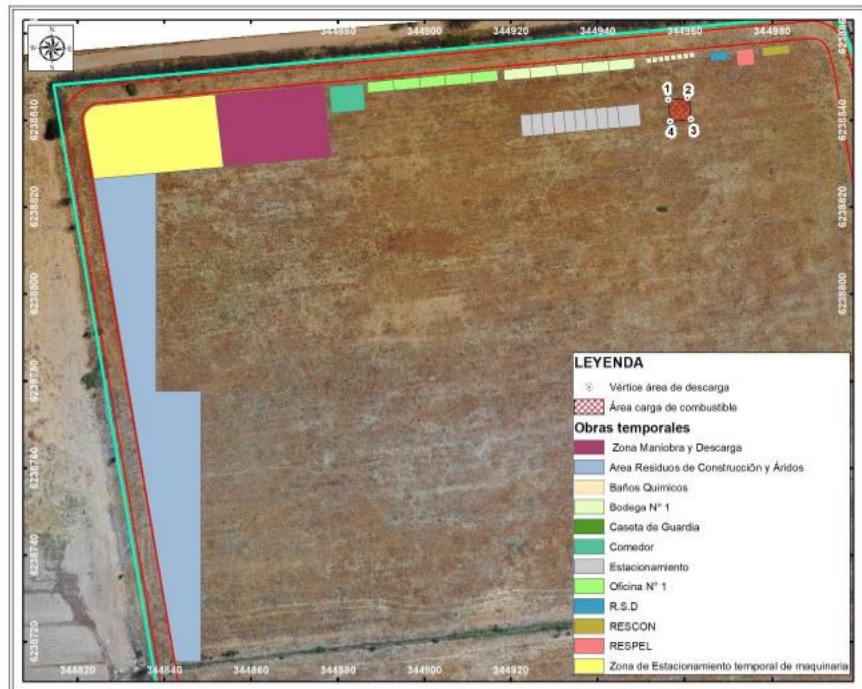
Figura 1-40. Área destinada a la carga de combustible del grupo electrógeno.
