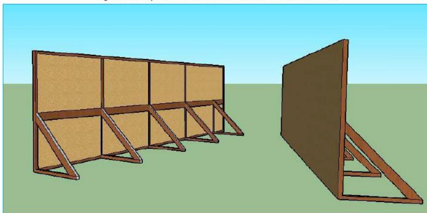
Figura 24: Esquema de barrera acústica modular trasladable,
