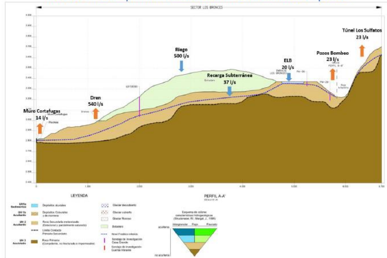
FIGURA C4-13: Esquema del balance hídrico en la cuenca La Disputada
