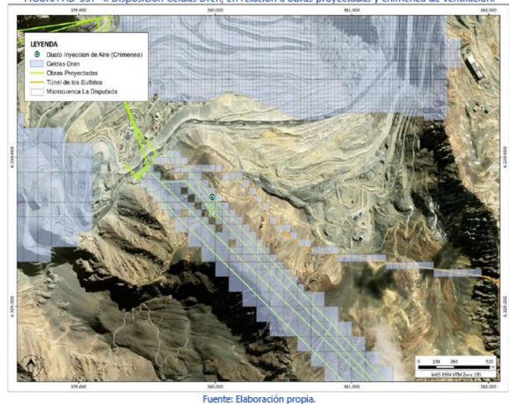
FIGURA AD-557-4: Disposición Celdas Dren, en relación a obras proyectadas y chimenea de ventilación.
