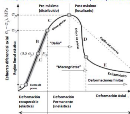
FIGURA ADC-234-1: Etapas teóricas de deformación que se producen en el macizo rocoso.
