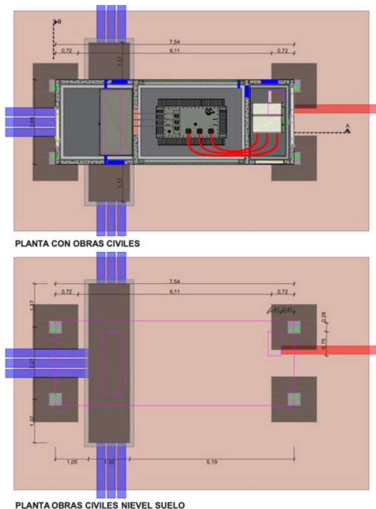
PLANTA OBRAS CIVILES NIVEL SUELO
