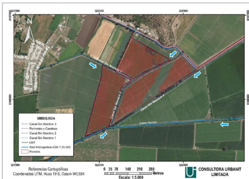
Figura 3-4. Red Local de Canales
