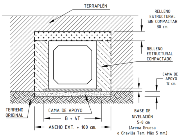
Cajones prefabricados de hormigón armado según Manual de Carreteras Vol 4, 2018
