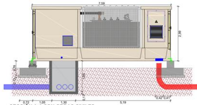
SECCIÓN A-A CON OBRAS CIVILES
