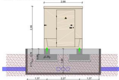
SECCIÓN B-B CON OBRAS CIVILES
