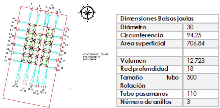
Figura 16. Disposición general de las balsas jaulas y fondeos del proyecto.
