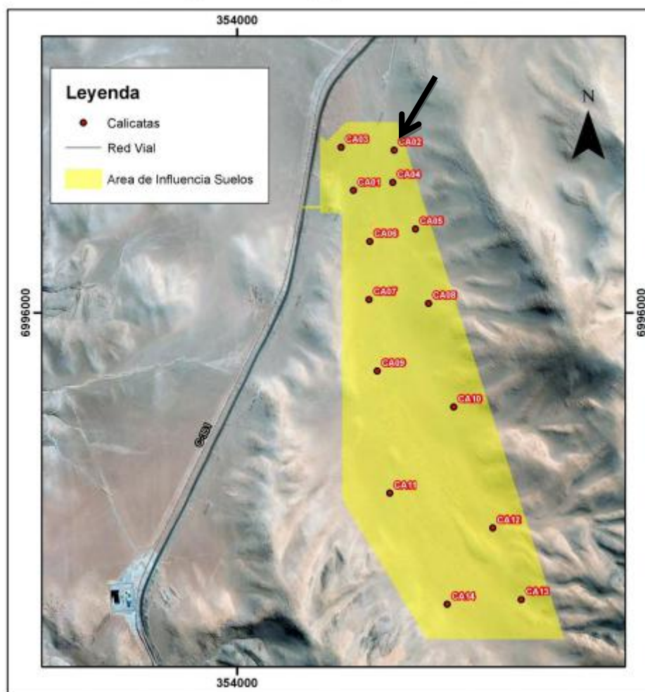
Figura N° 6. Calicatas (CA) realizadas en terreno.
