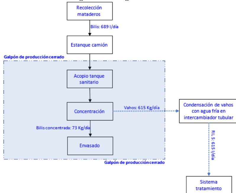
Imagen N°7. Diagrama línea bilis
