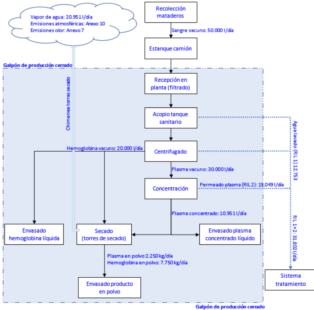
Imagen N°5. Diagrama proceso línea
